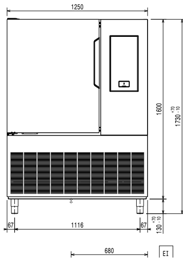
Alzado
