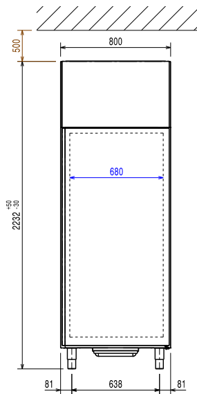
Alzado
